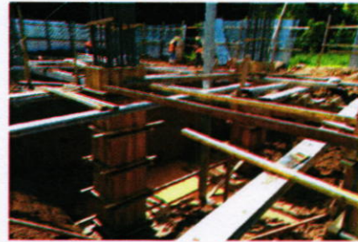
Encofrado de Pedestales de concreto (Grupo Nor-Oeste). 31-01-2017
