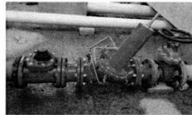
Medidor de caudal, Valvula de control de nivel de agua con piloto de altitud y Valvula de control de flujo de entrada de agua al tanque; 15-08-2018
