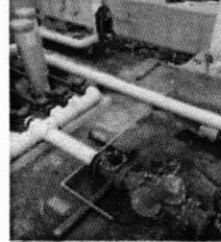
Medidor de caudal, Valvula de control de nivel de agua con piloto de altitud y Valvula de control de flujo de entrada de agua al tanque; 30-09-2018
