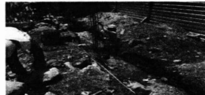
Armado de hierro y encofrado de zapatas aisladas de 80x80x25cms en el sector oeste.
