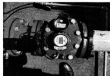
Medidor de caudal de 6"Ø instalado en la tubería de entrada al tanque; 30-10-2018
