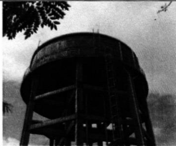
Vista General del Tanque Elevado; 30-10-2018
