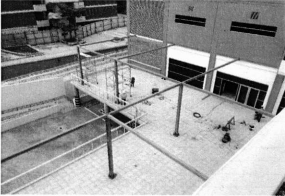
Instalación de estructura metálica de pérgolas en terraza de Comedor.
