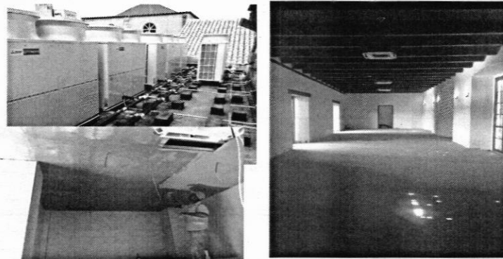
Se continua trabajando en las instalaciones del sistemas Electrico, Mecanico, de aire acondicionado, terminando de instalar la ducteria, las unidades caseth, cableado para lamparas, etc. y tambien los acabados de la cafeteria.
