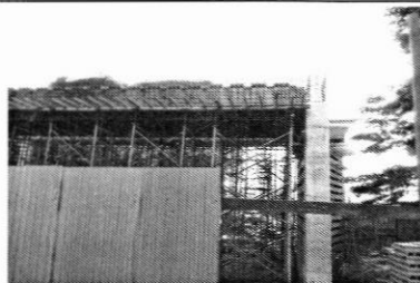
Instalación de vigueta y bovedilla en losa de techo portal peatonal
