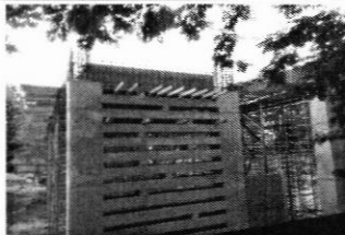
Avance en encofrado de losa y armado de viga perimetral en techo de portal peatonal
